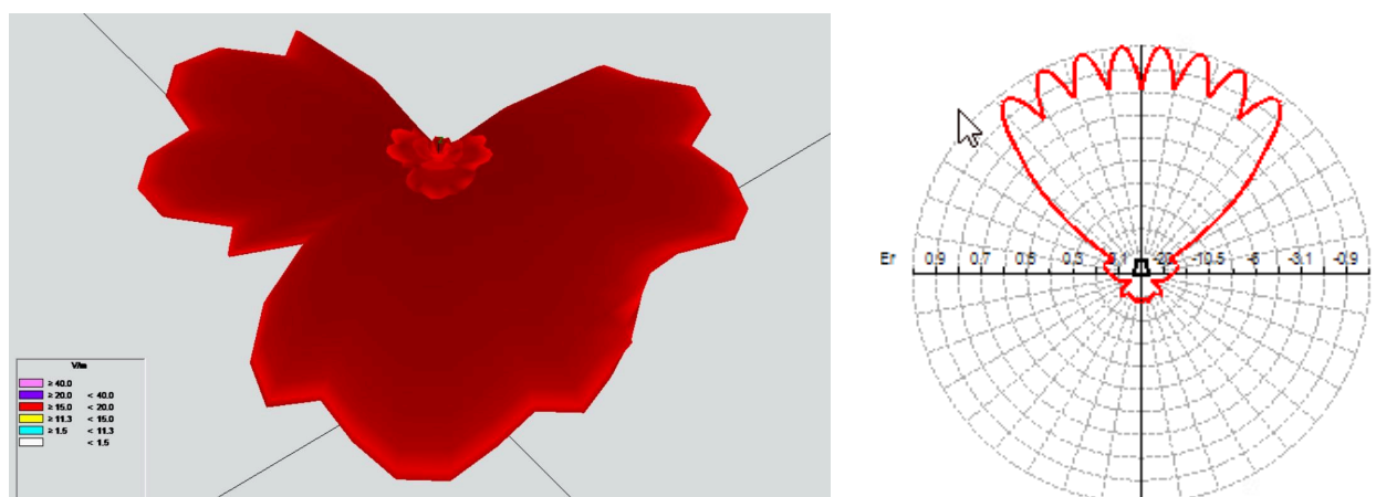
Figura 7: isovolume a 15 V/m generato da tre sistemi d'antenna con tecnologia 5G -3700 MHz utilizzando i fattori di correzione statistici (a sinistra); diagramma orizzontale a involuppo di un'antenna massive MIMO (a destra).
