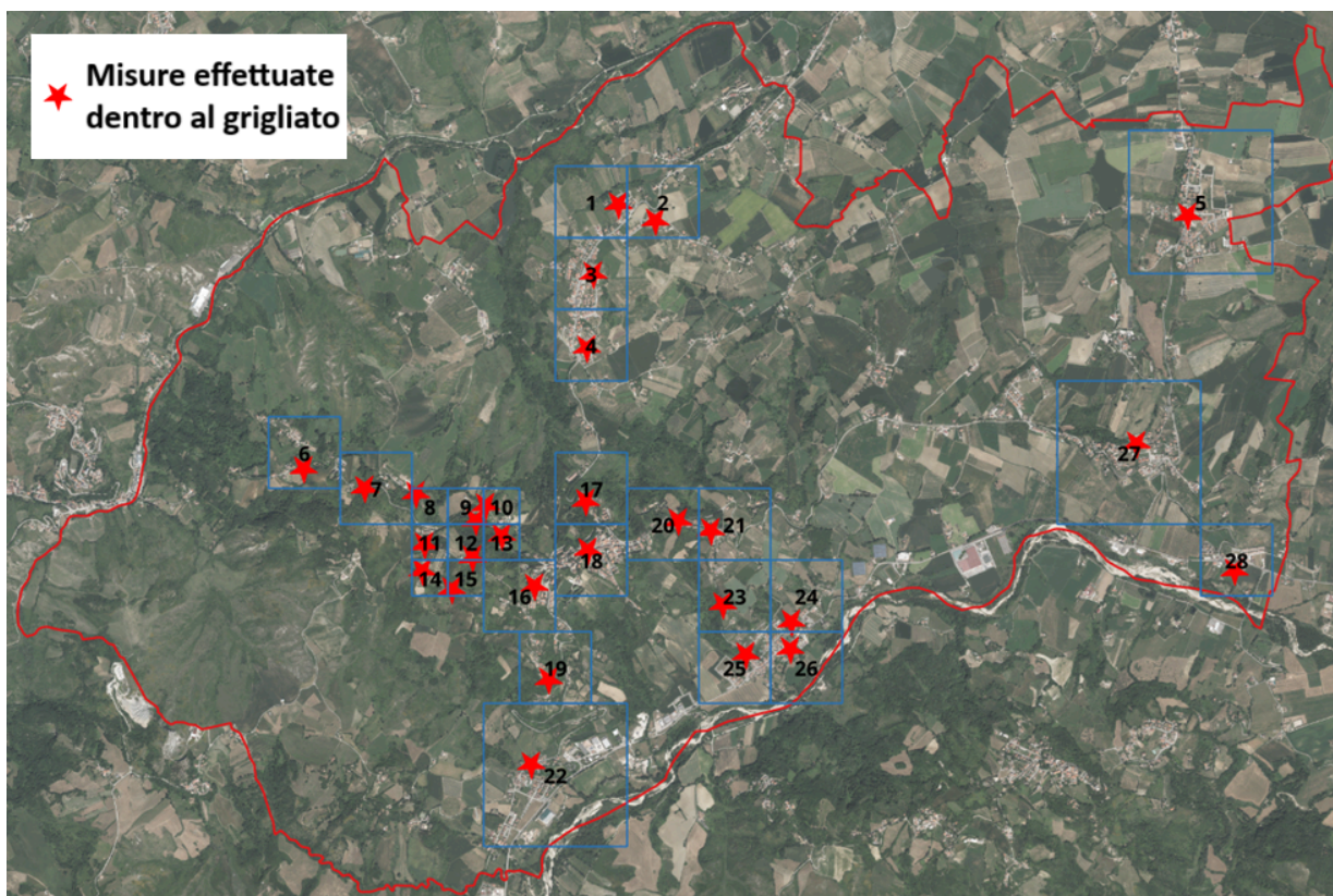
Figura 11: rappresentazione dei punti di misura del campo elettrico RF all'interno del grigliato
