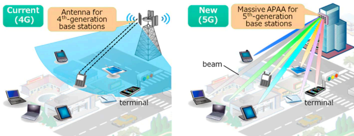
Figura 6: il beamforming implementato nella tecnologia 5G
