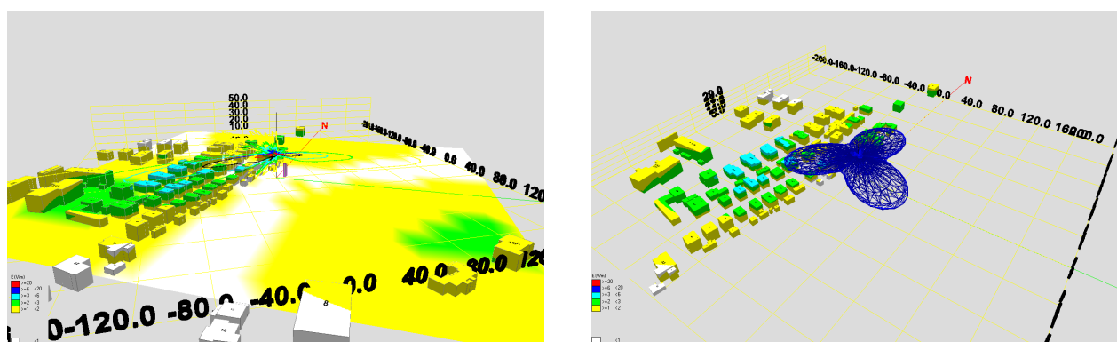
Simulazioni in 3D del Campo Elettrico (E) [V/m] generato da una SRB al suolo (a sinistra) ed in quota (a destra)
